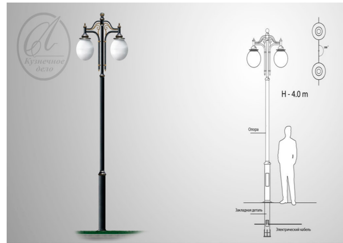
T/X по теме: Фонарь Павел 2. H - 4.0 м. Грунт: - Эмаль 3в1 (антикоррозийный). Электрокомплектация: Для индивидуального подхода по теме T/X Опора: Сталь - (С15ПС, 08ПС). Краска: Forgent Paint (Черный). Е 27. контакт с производством Рассеиватель: Шар 400. Патина: WS - Patina (под Золото). ПВС 3Х1.5. тел. факс: (8652) 23 04 81. (Полим Сталь - (С15ПС, 08ПС). ЗНИ -16. (8652) 22 04 41.
